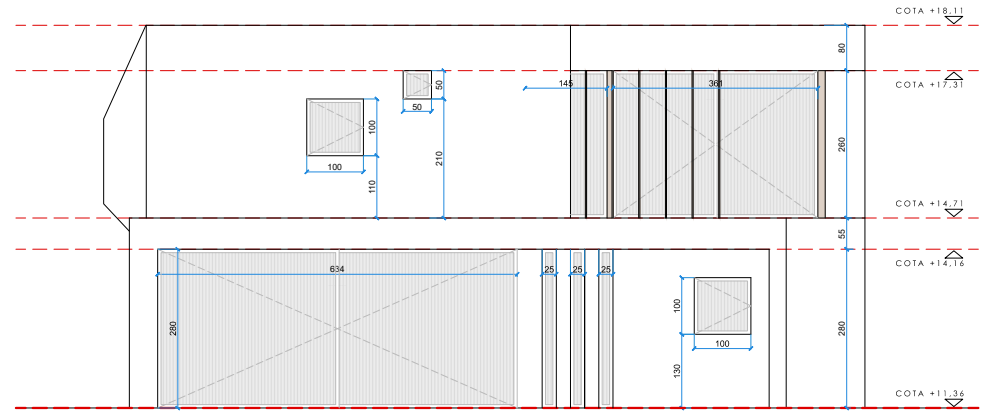
ALZADO OESTE
