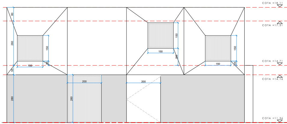
ALZADO NORTE
