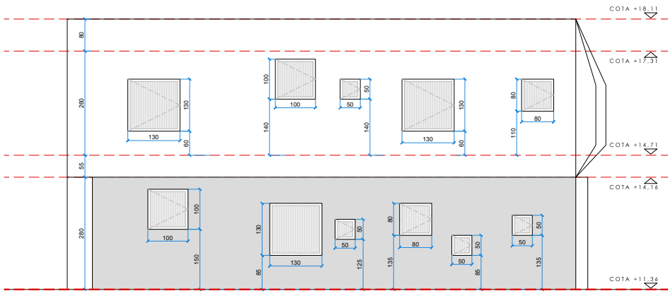
ALZADO ESTE
