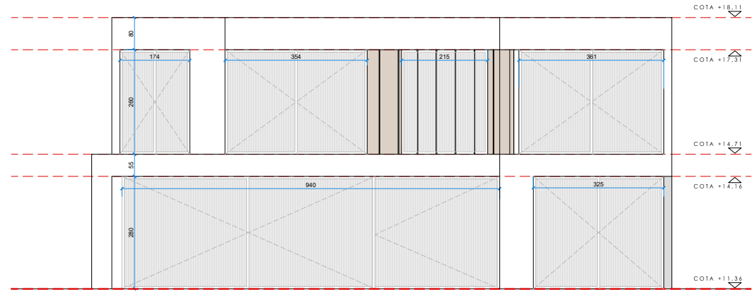
ALZADO SUR
